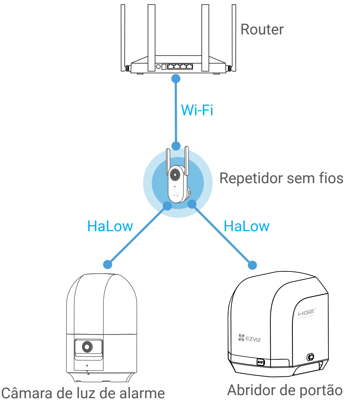
Topologia de comunicação sem fios
